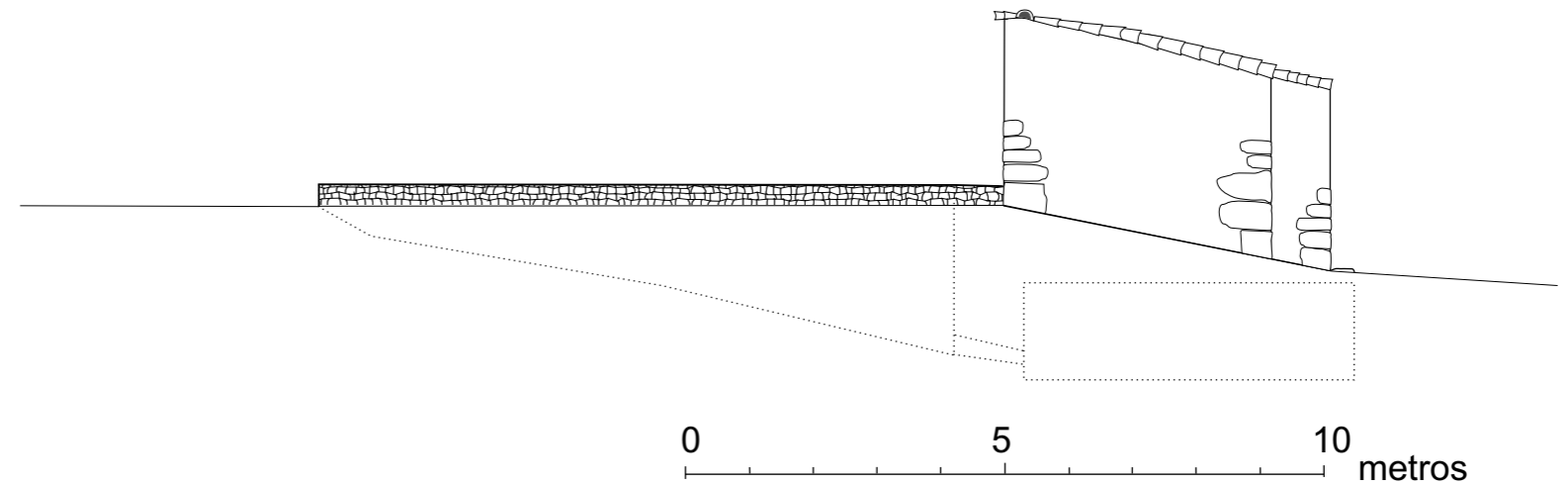
Alzado Suroeste
